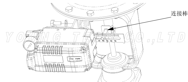
图：阀杆连接件和反馈杆连接
