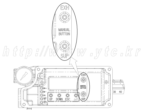
图：手动旋钮
