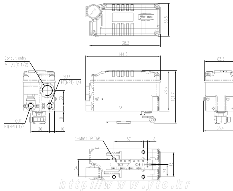
图：YT-2700L 外形图
