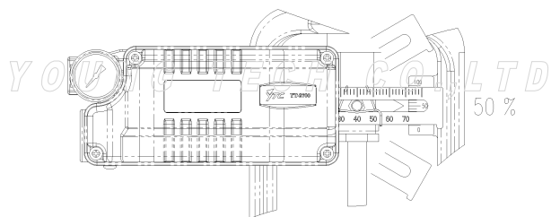
图：反馈杆正确成水平的状态图
