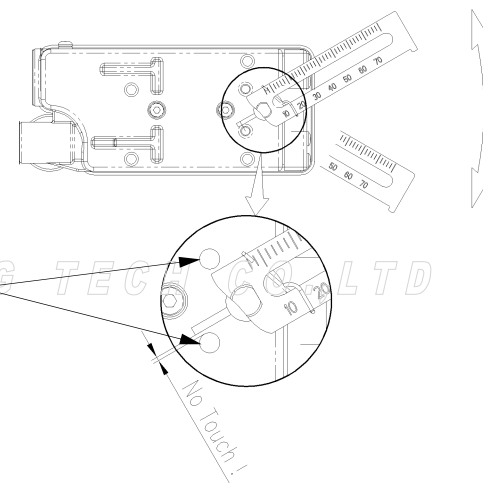
图：反馈挡板和反馈杆之间非接触的状态图
