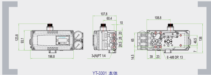
YT-3301 本体
