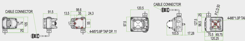
YT-3301L 传感器
