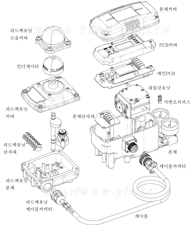
그림 : YT-2501R 전체 구조도
