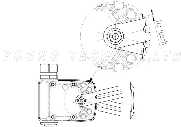
그림 : 레버스토퍼와 피드백레버의 비접촉상태 확인
