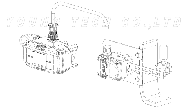
그림 : YT-2501L 설치 상태 예
