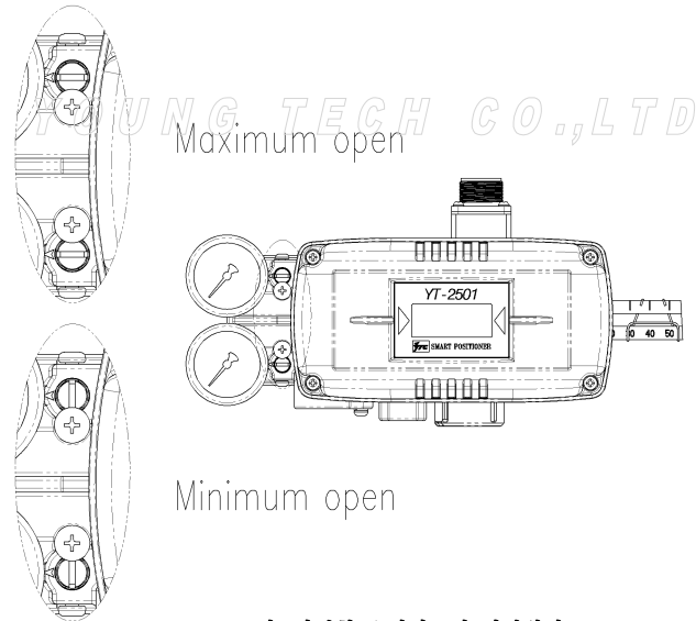
그림: 가변형 오리피스스의 회전위치
