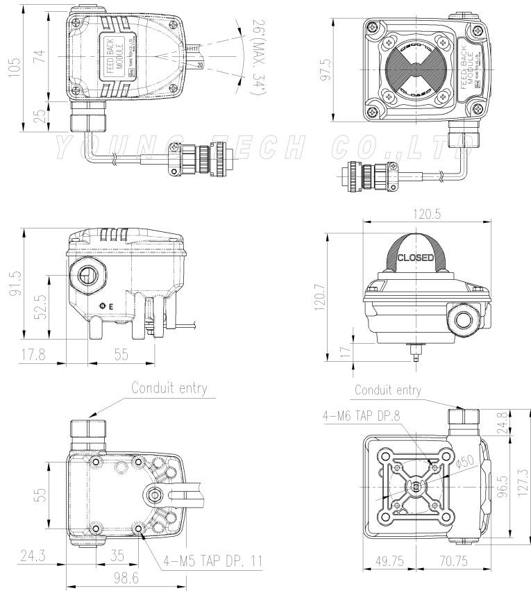
<YT-2501L Type> <YT-2501R Type>
