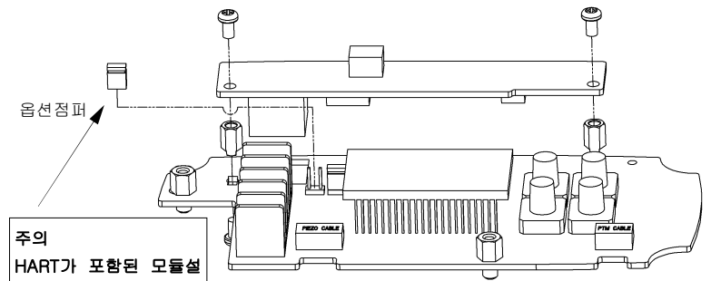
그림: 옵션기판의 설치 방법
