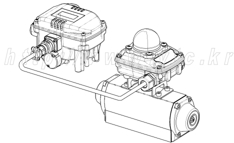
그림: YT-2501R의 설치 예
