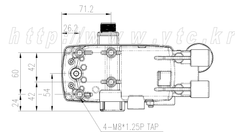
그림 : YT-2501 본체 외형도
