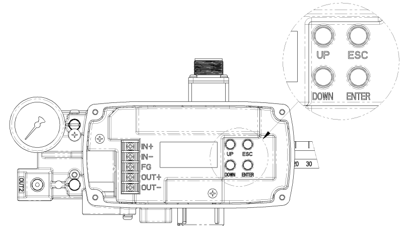
그림. YT-2501의 커버를 연 상태에서 위에서 본 그림
