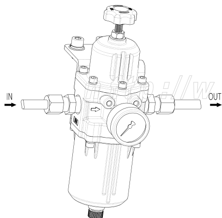
< 배관을 이용한 설치 예 >
