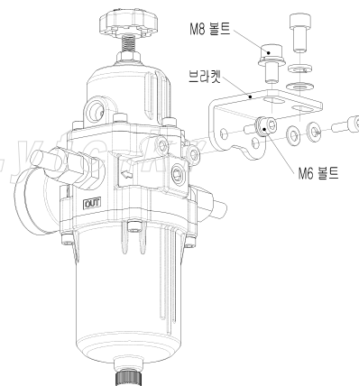
< 브라켓을 이용한 설치 예 >
