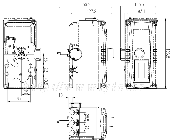
그림 : YT-3300R L/S 옵션 외형도
