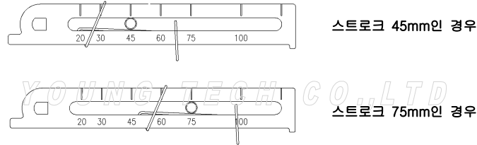
그림 : 밸브 스트로크에 대한 연결봉 설치 위치
