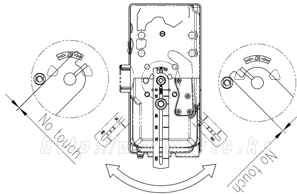
그림 : 레버스토퍼와 피드백레버의 비접촉상태 확인
