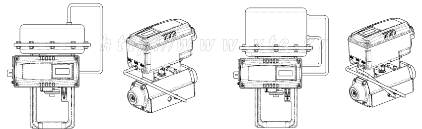
단동식 액츄에이터 공압배관 연결
