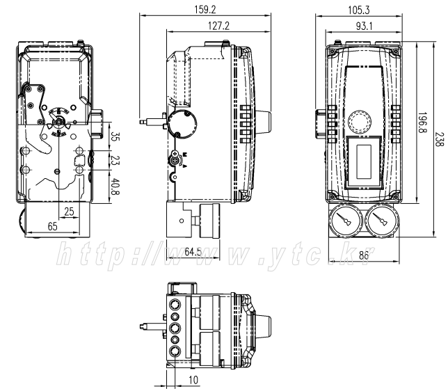
그림 : YT-3300R L/S & 2 게이지 옵션 외형도
