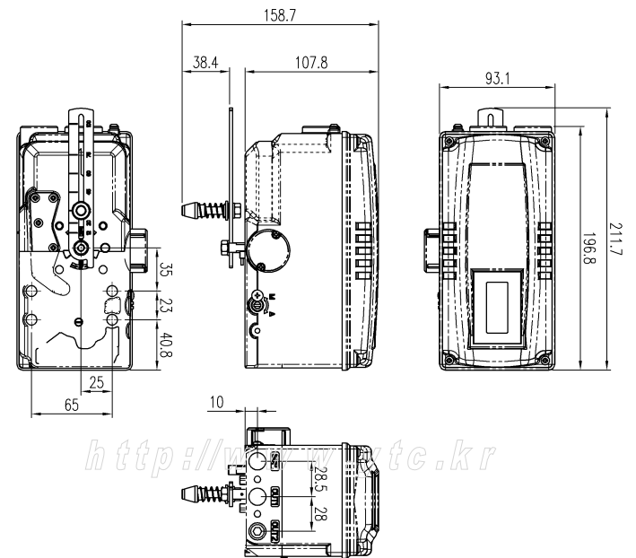
그림 : YT-3300L 외형도
