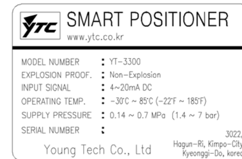
그림 : YT-3300 라벨
