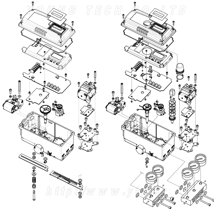
그림 : YT-3300L 구조도
