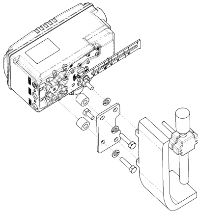
그림 : YT-3300L과 브라켓 조립하기
