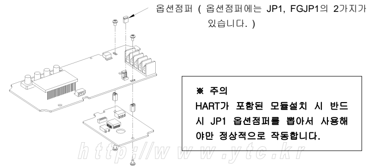
그림: 옵션기판의 설치 방법
