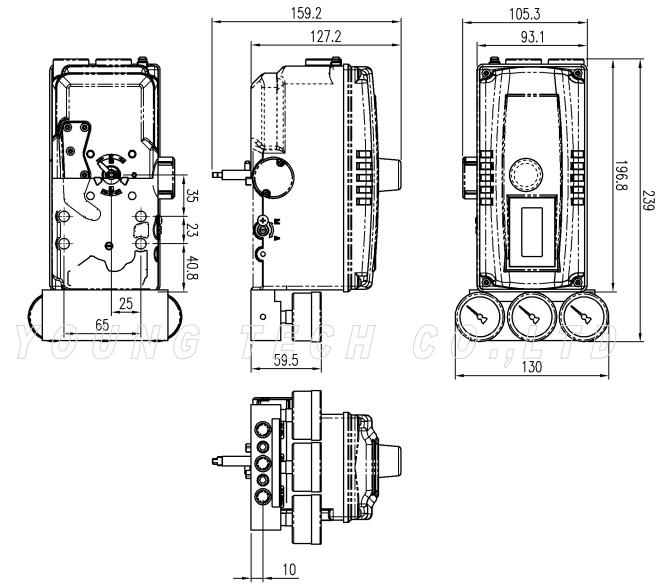
그림 : YT-3300R L/S & 3게이지 옵션 외형도
