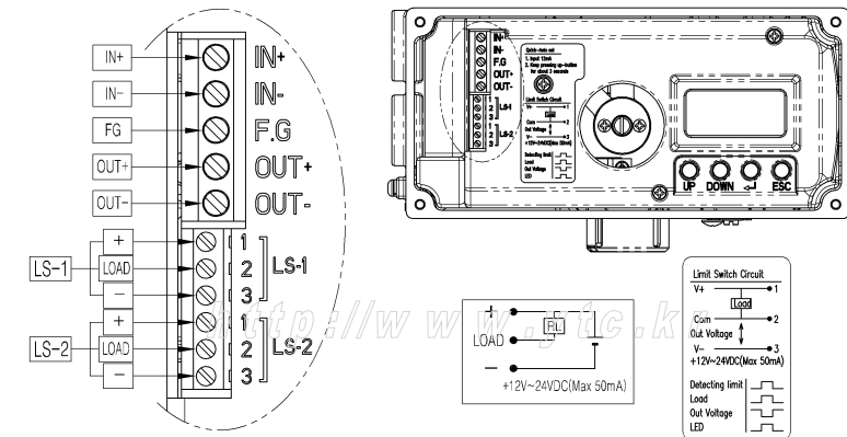
그림: 비접촉식 스위치 장착시
