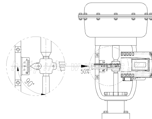
그림 : 피드백레버가 바르게 수평을 이룬 상태
