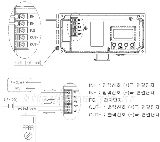
그림 : 전류입력신호 및 피드백신호의 연결
