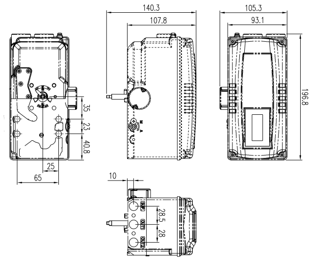
그림 : YT-3300R 기본형 외형도
