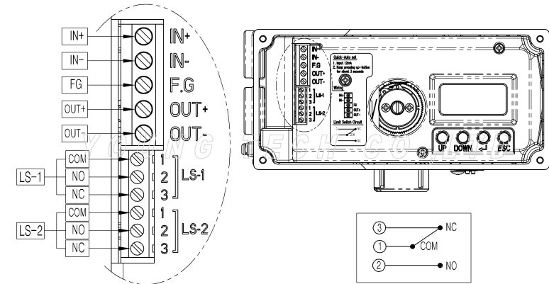
그림: 마이크로 스위치 장착시
